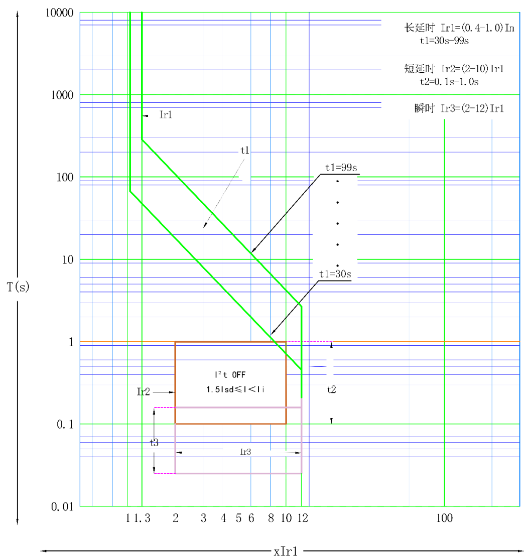
时间/电流特性曲线图
