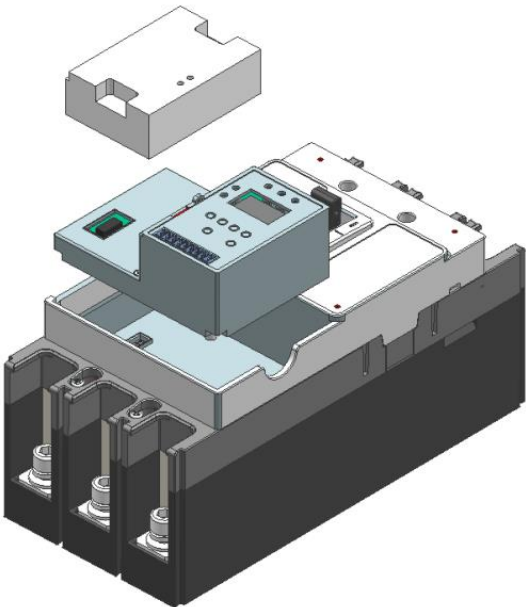
控制模块分离示意图
